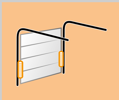
Kovanie Z: Kovanie s ťažnými pružinami s technikou ťažných pružín
