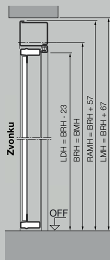
Vertikálny rez dverí bez dolného dorazu
