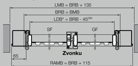
Horizontálny rez
