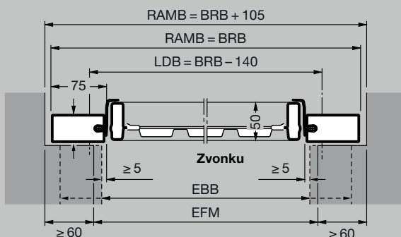
Horizontálny rez – montáž za otvor
