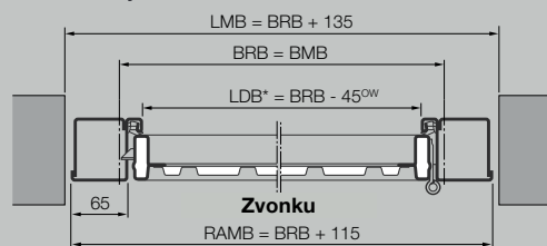
Horizontálny rez
