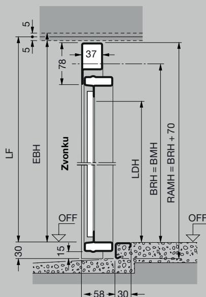
Vertikálny rez brána s dolným dorazom
