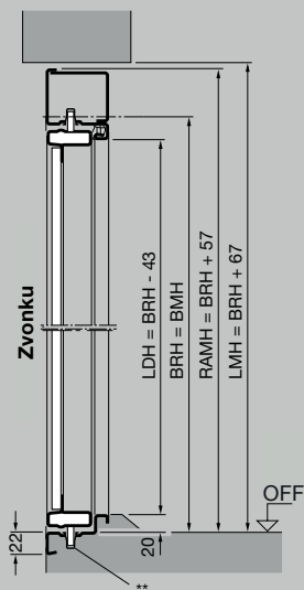
Vertikálny rez dverí s dolným dorazom
