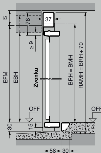
Vertikálny rez brána s dolným dorazom
